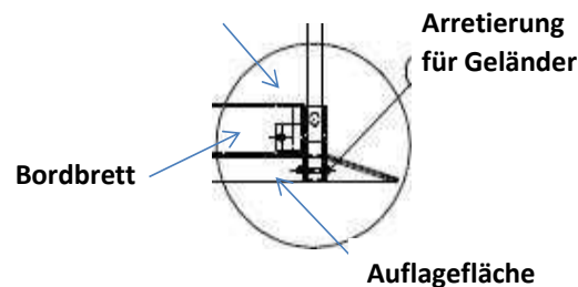
Auflagewinkel zum Stapeln
