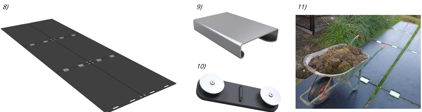
Abb. 8: Platten verbunden mit Schnell- und Einzelverbindern Abb. 9: Schnellverbinder 33901-1 Abb. 10: Einzelverbinder 33901-2 Abb. 11: Anwendung mit Schnellverbindern verbundener Platten
